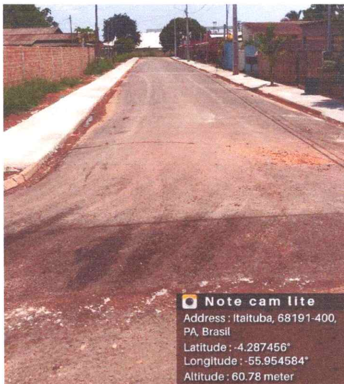
FOTO 2: PAVIMENTAÇÃO, MEIO FIO COM SARGETA E CALÇADA FINALZADOS
