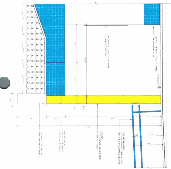
AMPLIAÇÃO FACHADA - ACESSO PRINCIPAL
